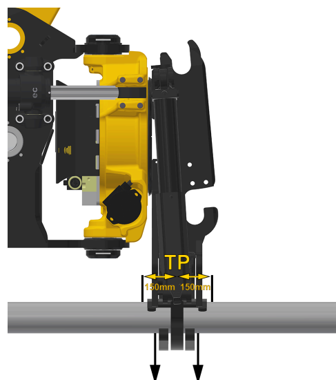
Afbeelding36. Maximale zwaartepuntverschuiving 150mm
