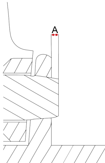
Werktuigbevestiging HS
